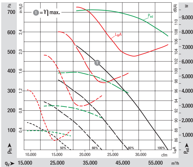
EC-Mitteldruck-Axialventilator Baugröße 1120
