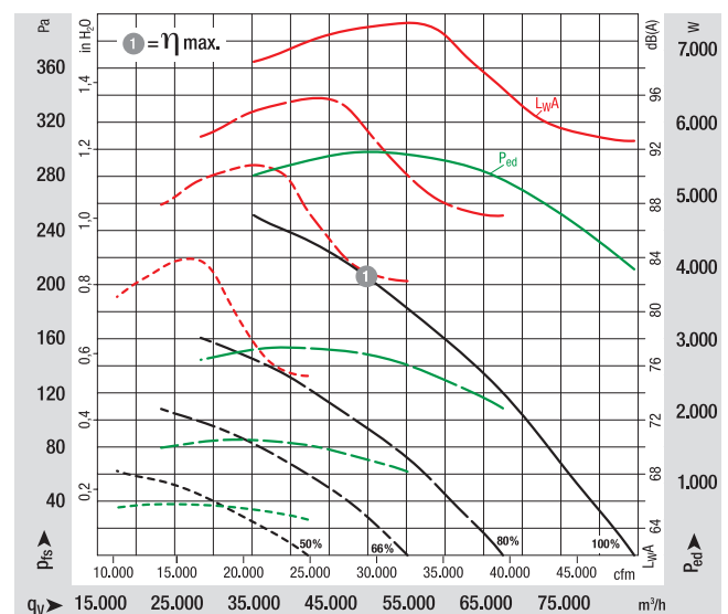
EC-Mitteldruck-Axialventilator Baugröße 1600
