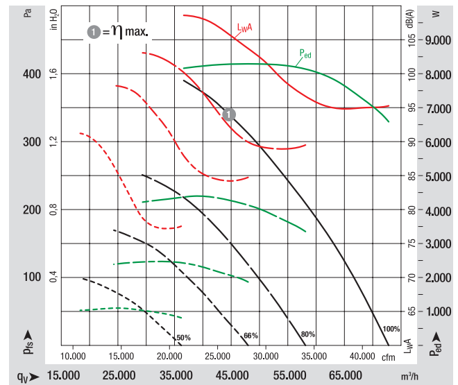
EC-Mitteldruck-Axialventilator Baugröße 1250
