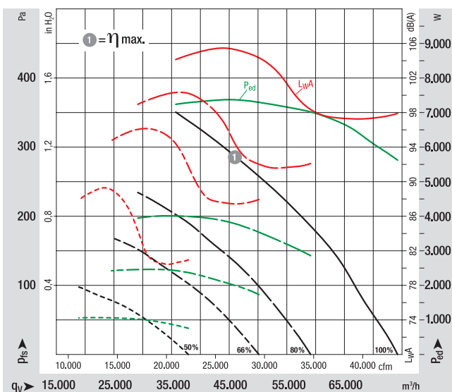
EC-Mitteldruck-Axialventilator Baugröße 1400
